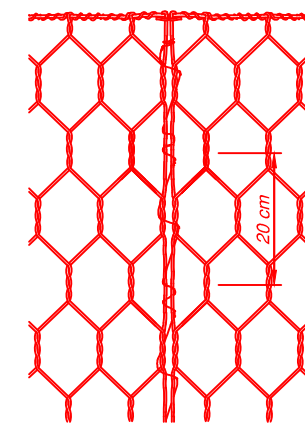
Detalhe da Costura
