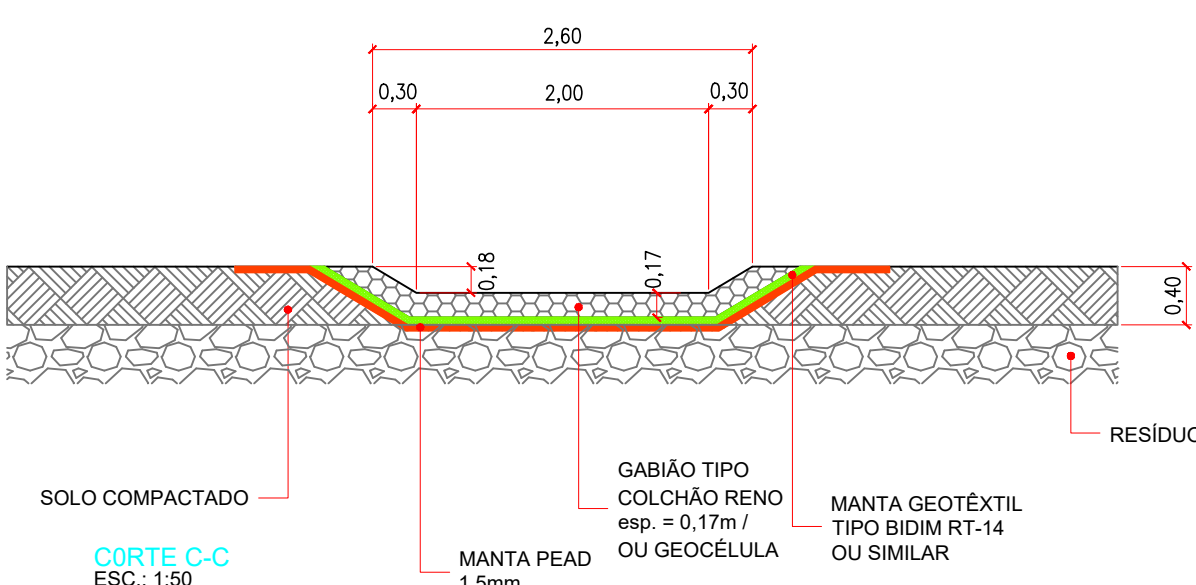
CORTE C-C ESC.: 1:50
