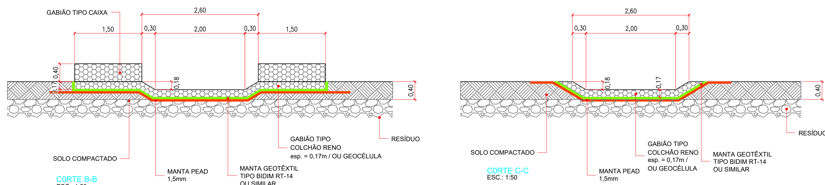
CORTE B-B ESC.: 1:50
