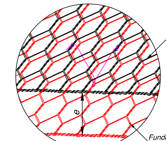
Detalhe (Colchão Reno®)
