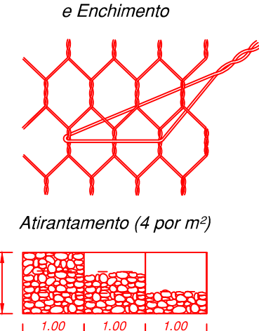
Detalhe do Atriantamento e Enchimento
