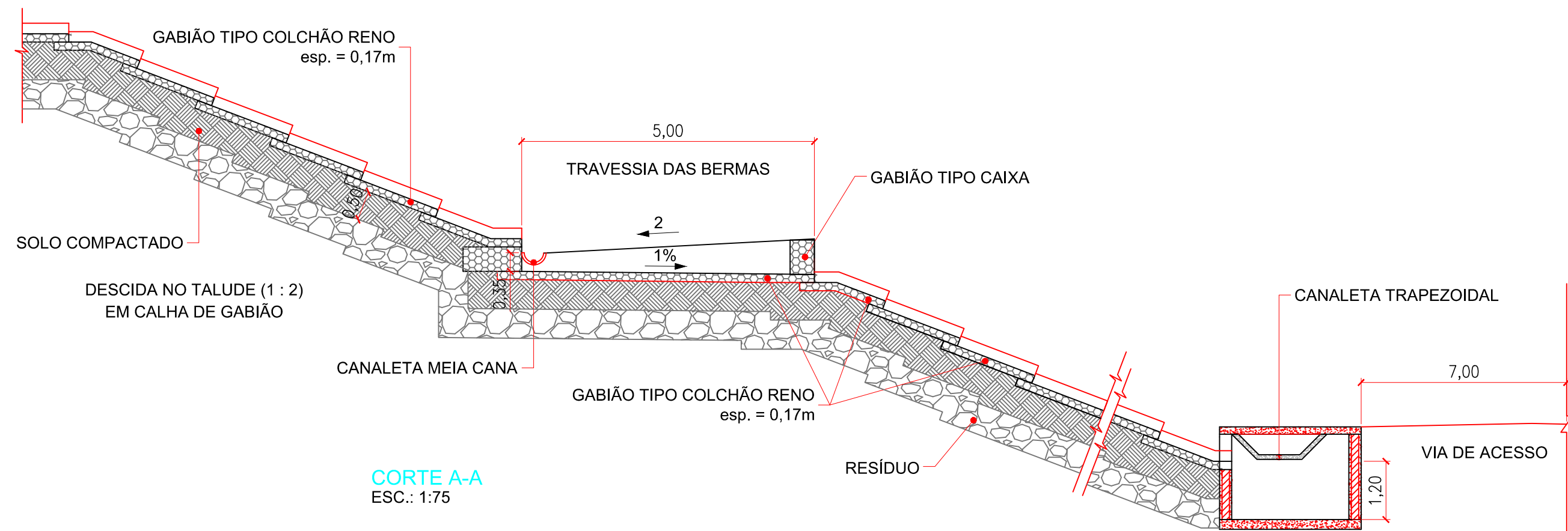
PLANTA ESC.: 1:75
