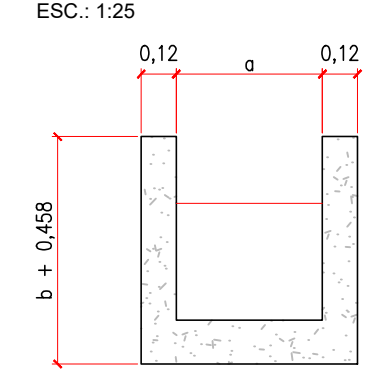
CORTE E-E ESC.: 1:25
