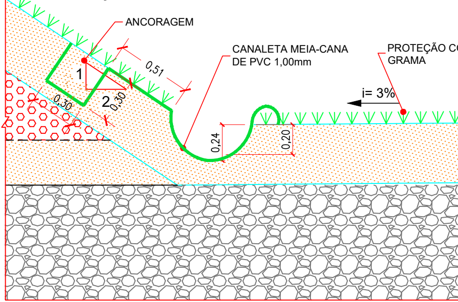
DETALHE TÍPICO DA CANALETA MEIA-CANA ESC.: 1:25
