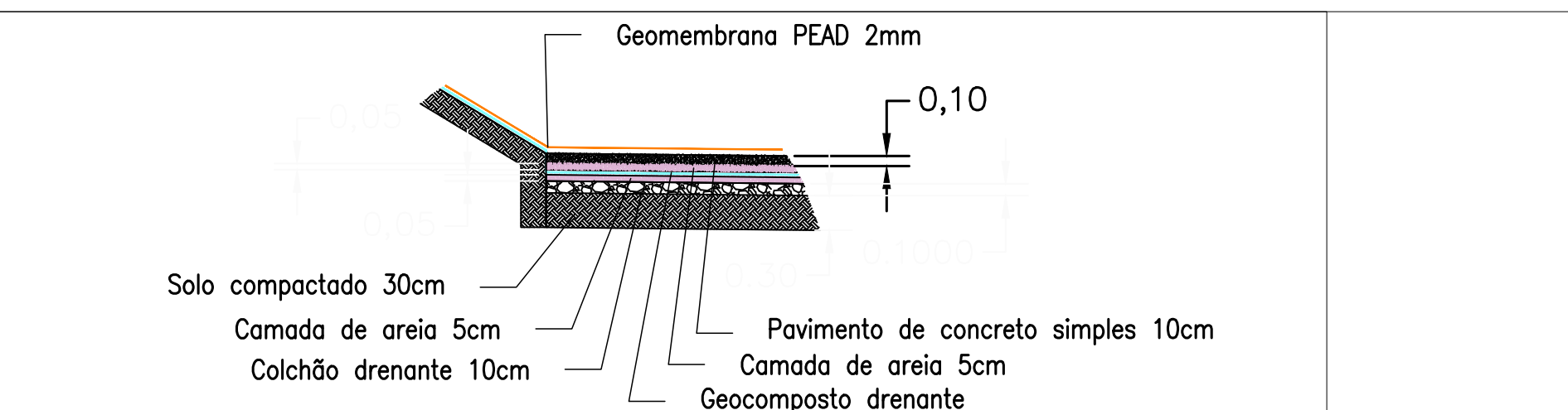
DETALHE DO COLCHÃO DRENANTE- RESERV. DE QUALIDADE 1 ESCALA - sem escala
