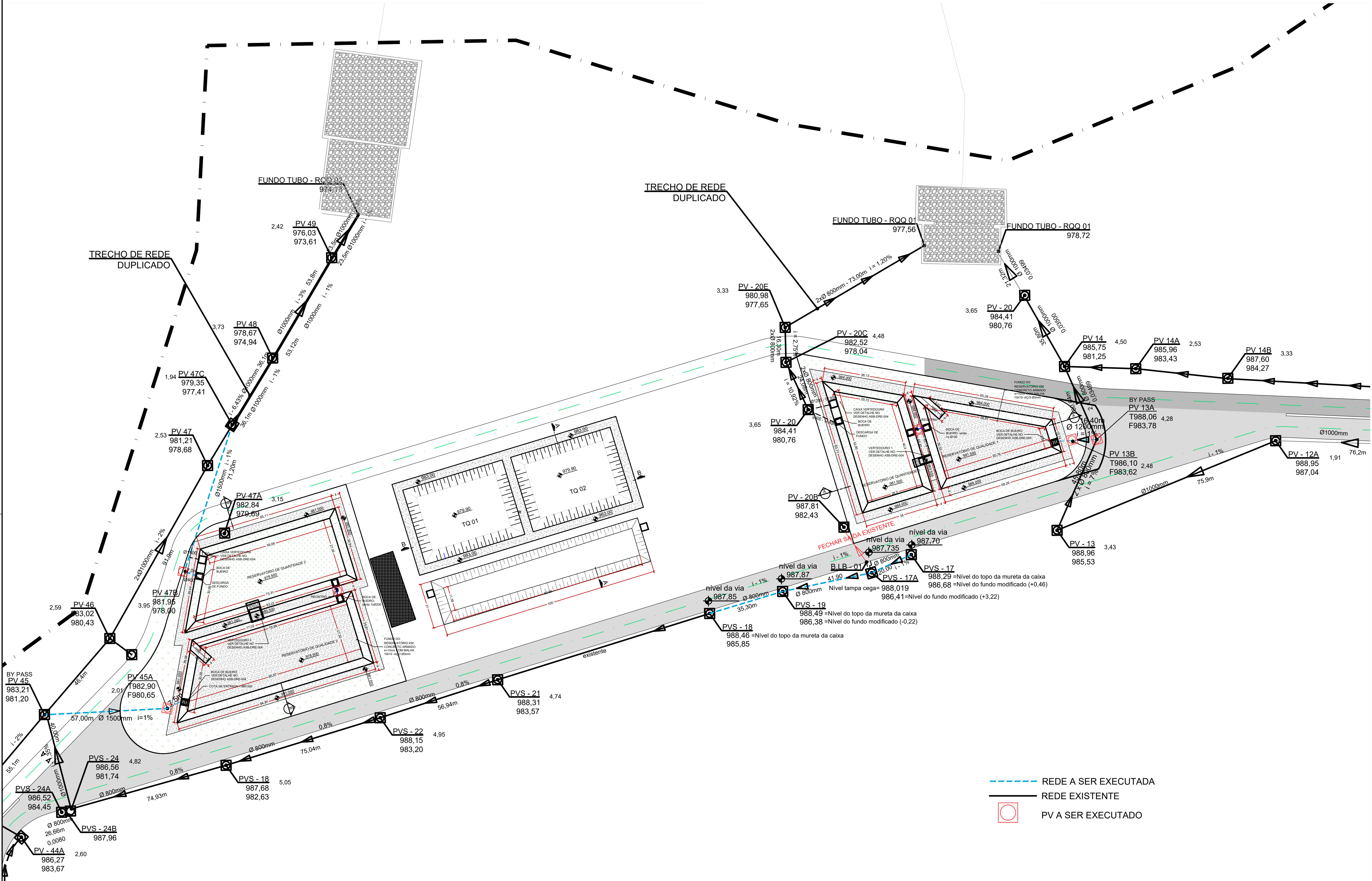
PLANTA BAIXA ESC 1:1000
