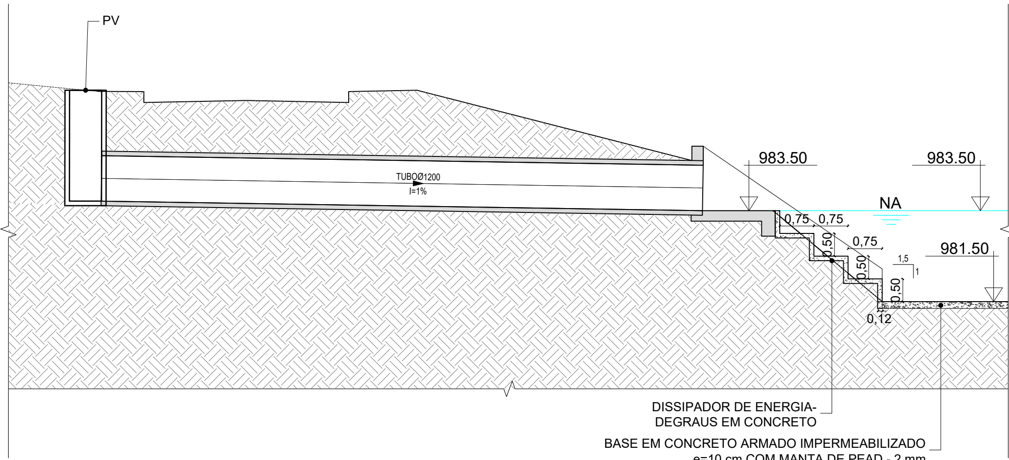
DETALHE DA ENTRADA DO RESERVATÓRIO DE QUALIDADE 1 ESCALA 1:75
