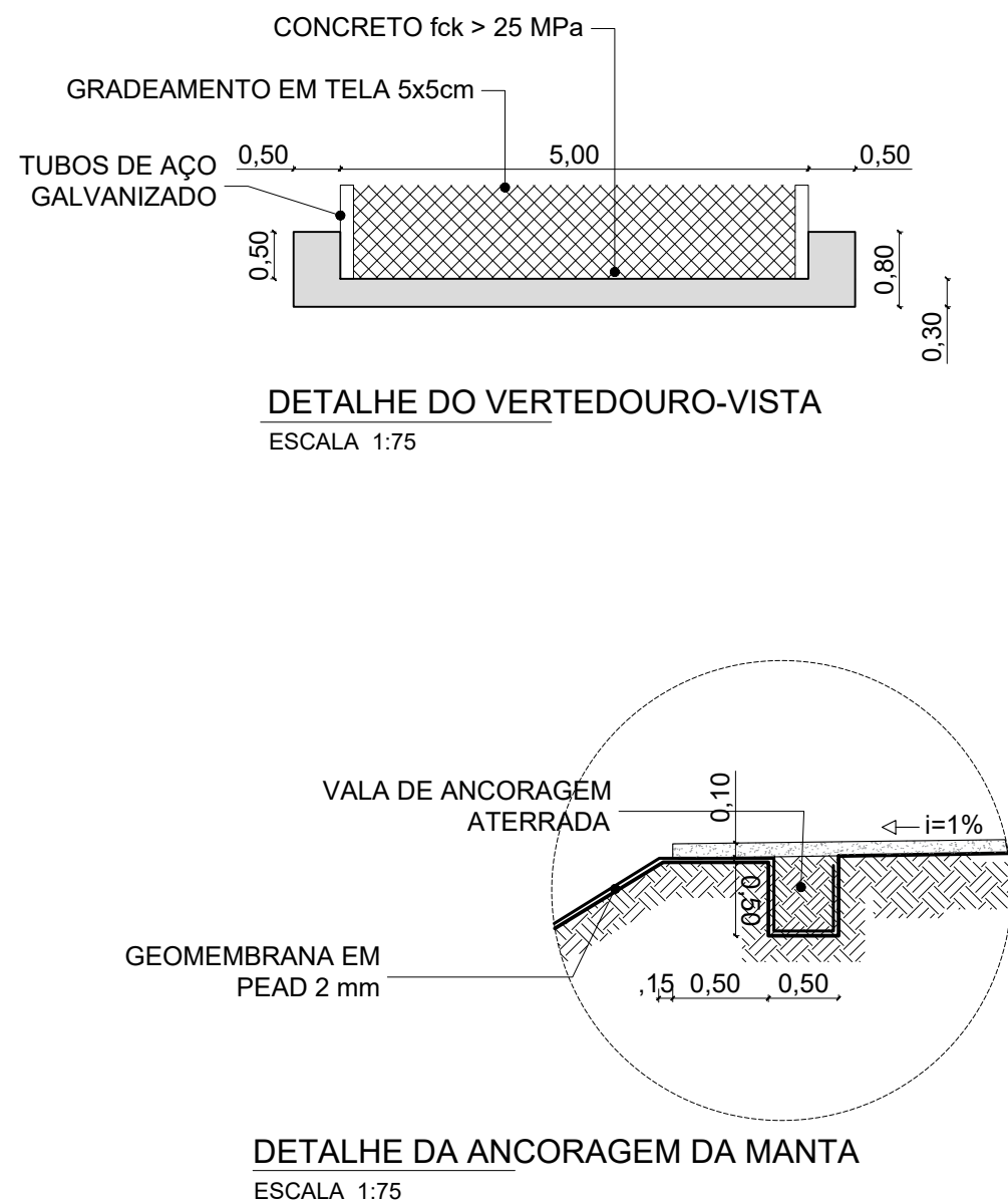
DETALHE DO VERTEDOURO 2-PLANTA ESCALA 1:75
