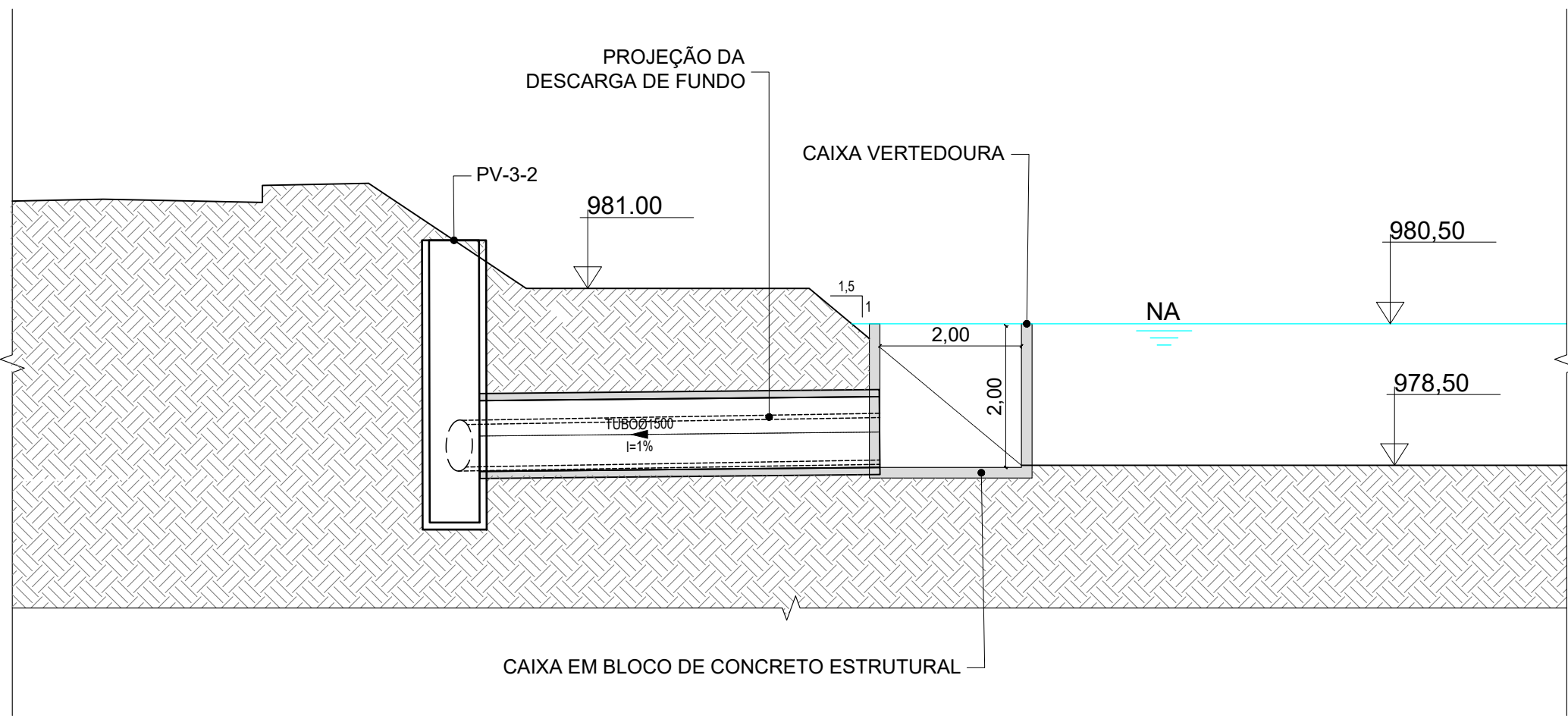
DETALHE DA SAÍDA DO RESERVATÓRIO DE QUANTIDADE 2 - CAIXA VERTEDOURA ESCALA 1:75
