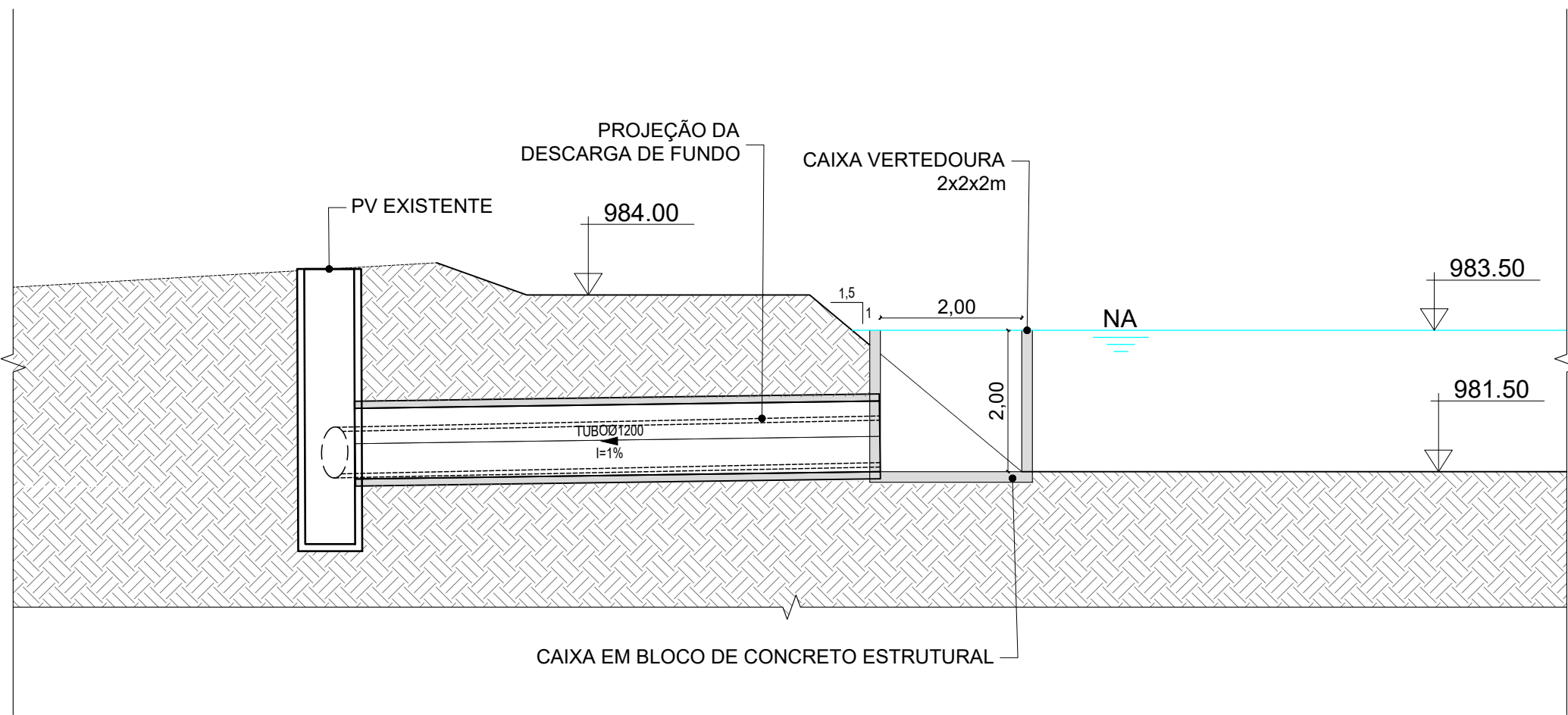
DETALHE DA SAÍDA DO RESERVATÓRIO DE QUANTIDADE 1 - CAIXA VERTEDOURA ESCALA 1:75
