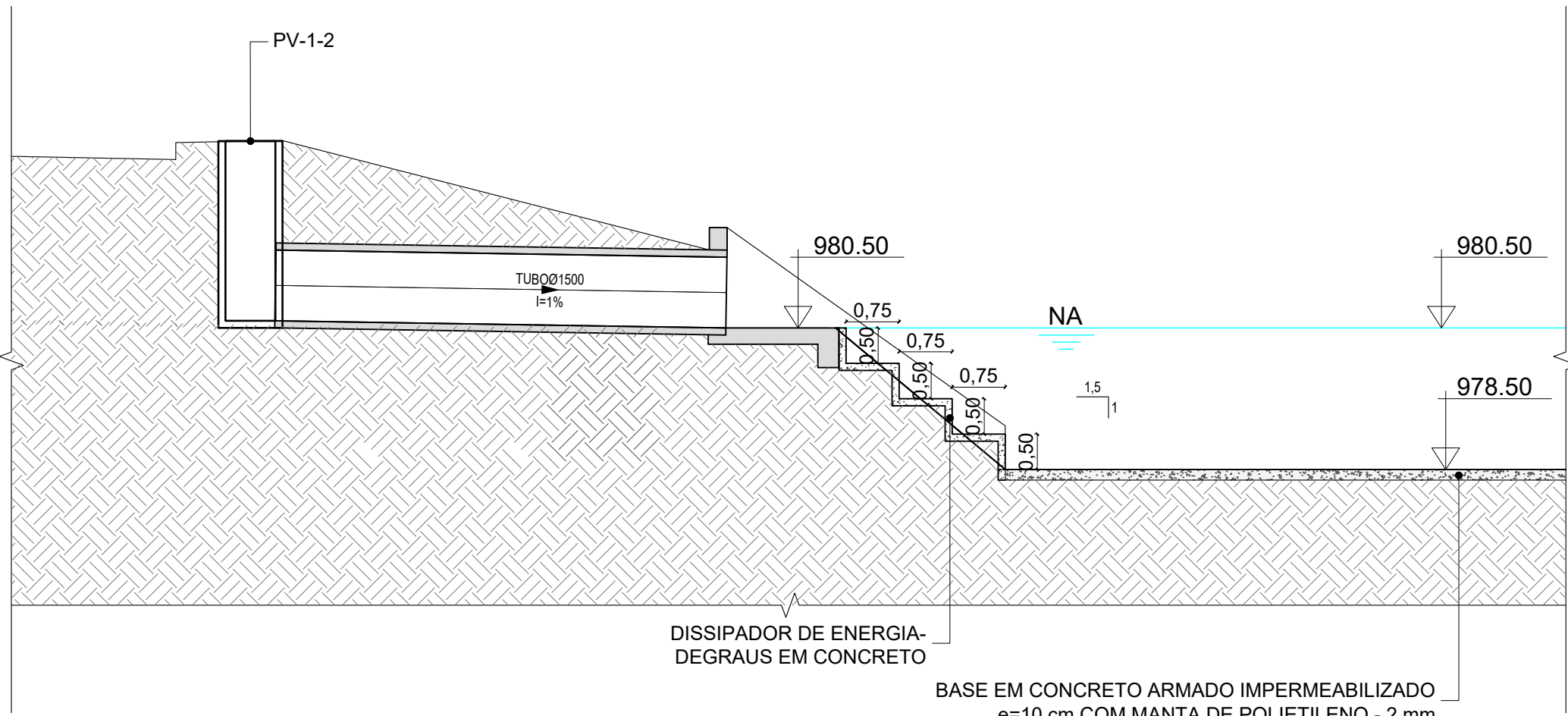
DETALHE DA ENTRADA DO RESERVATÓRIO DE QUALIDADE 2 ESCALA 1:75
