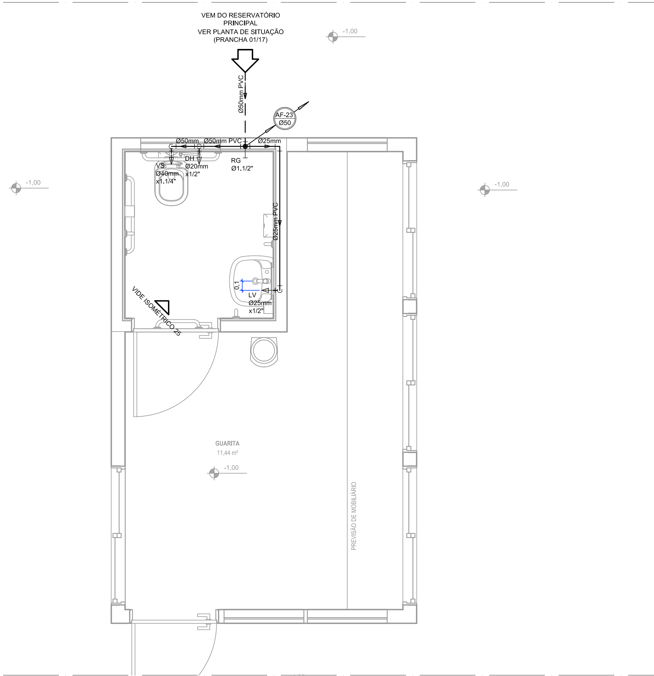
DETALHE 01 - PLANTA BAIXA DA GUARITA ESCALA 1:25
