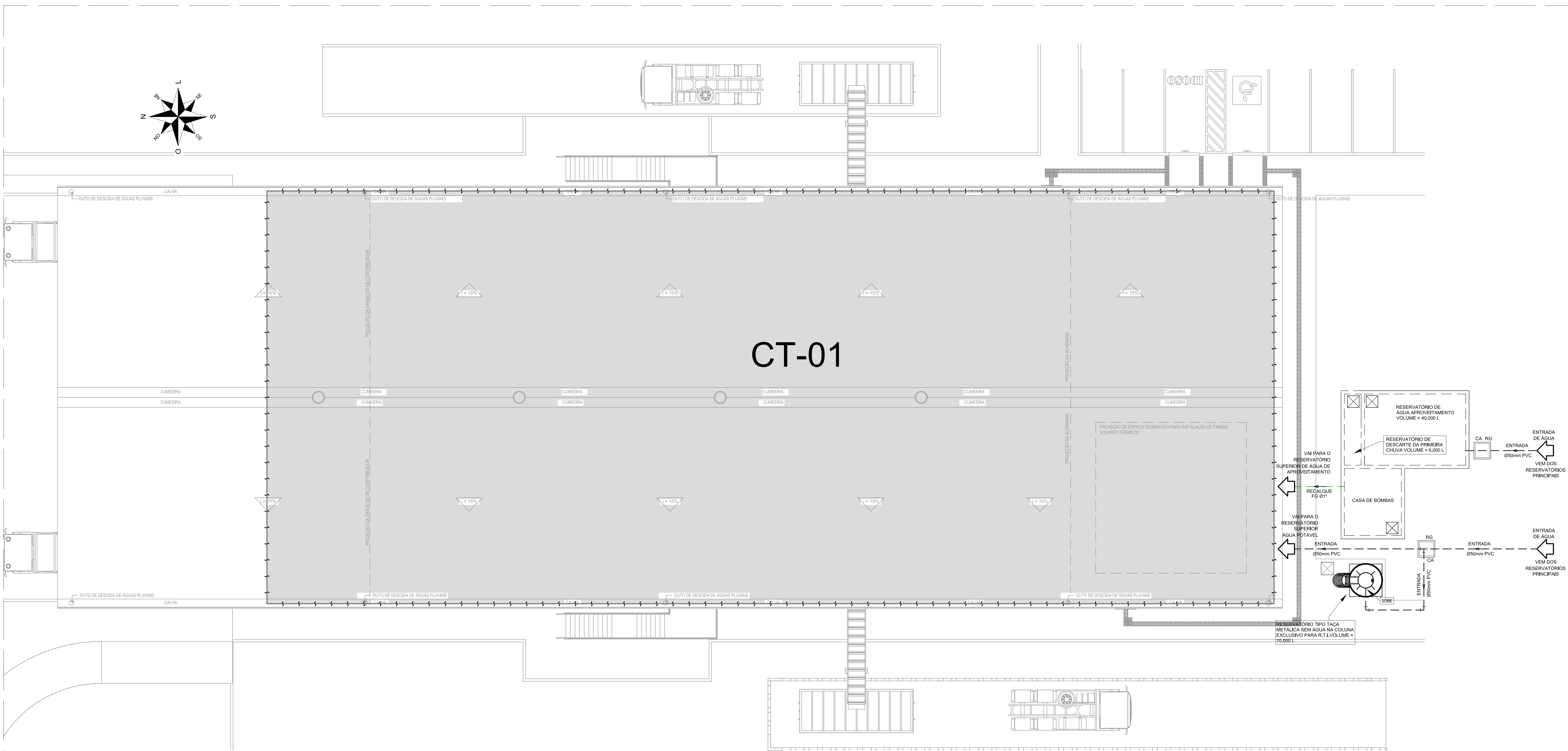
PLANTA DE IMPLANTAÇÃO - CENTRO DE TRIAGEM 01 ESCALA 1:100
