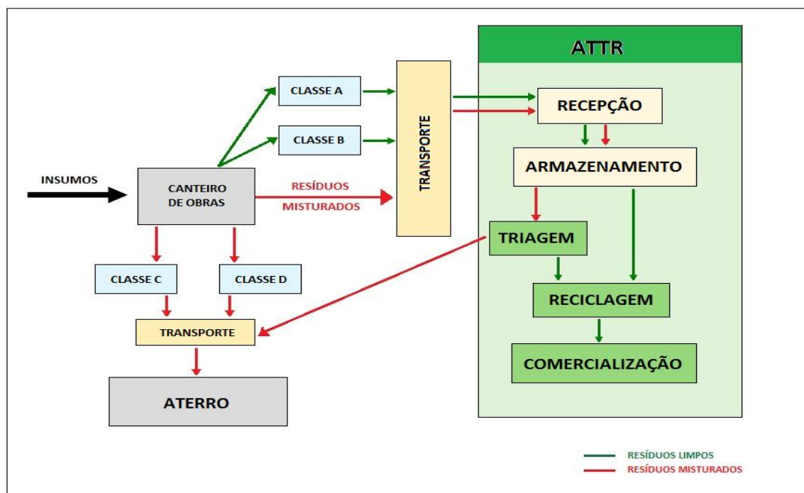
Figura 3: Logística de Funcionamento da Área de Transbordo, Triagem e Reciclagem
